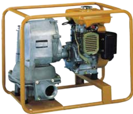
M 201 verpompt vaste bestanddelen tot 25mm
